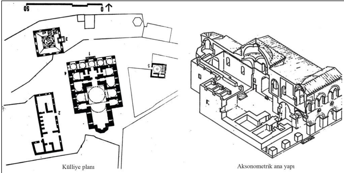
Zaviyeli Cami Plan Şeması K: www.sehrinesesver.com
